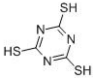
三聚硫氰酸
