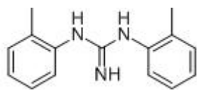
二邻甲苯胍
